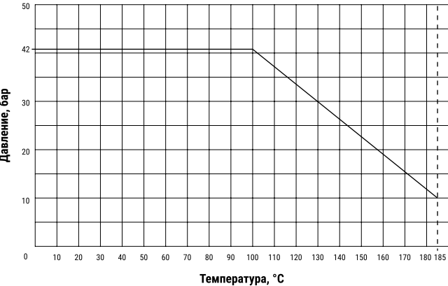
Зависимость рабочего давления от температуры перемещаемой среды.
